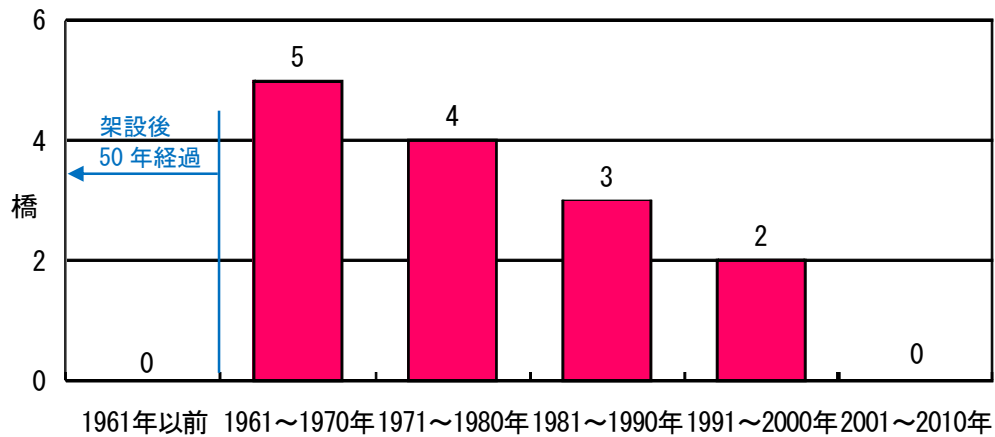
図-3.3 架設年次別の橋梁数
