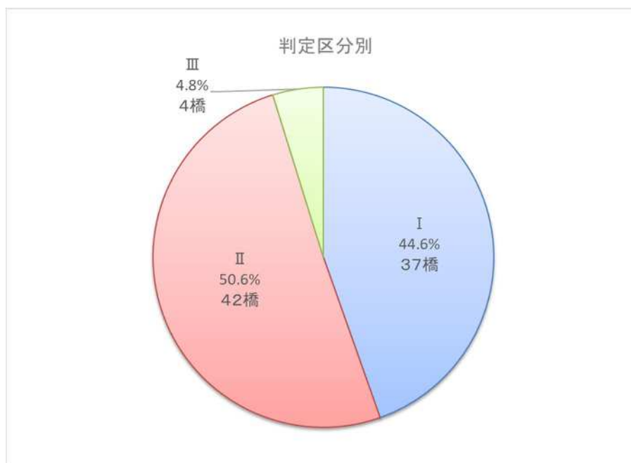
図 3-1 橋梁の健全度（令和6年度末時点）
