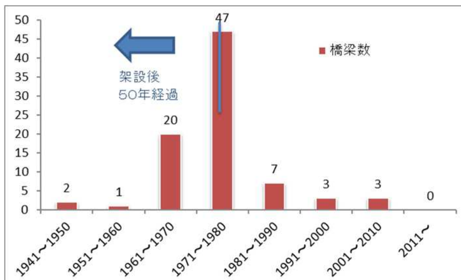
図 2-1 橋梁架設年次別の橋梁数（令和 6 年度末時点）
